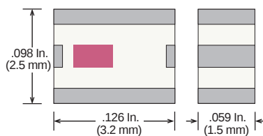
Case 41-1 (EIA 1210 / 3225)
