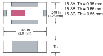
Case 15-3 (EIA 0805 / 2012)
