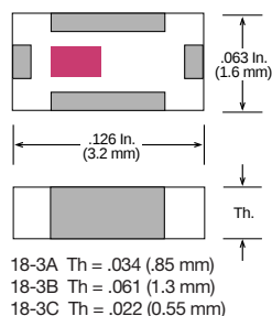
Case 18-3 (EIA 1206 / 3216)
